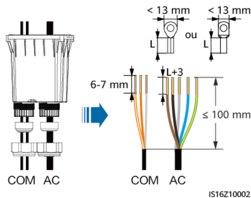
Figure 5-8 Acheminement des câbles
