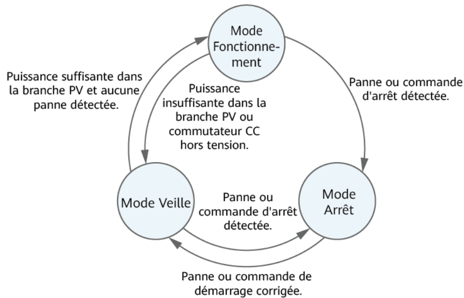
Figure 2-5 Modes de fonctionnement
