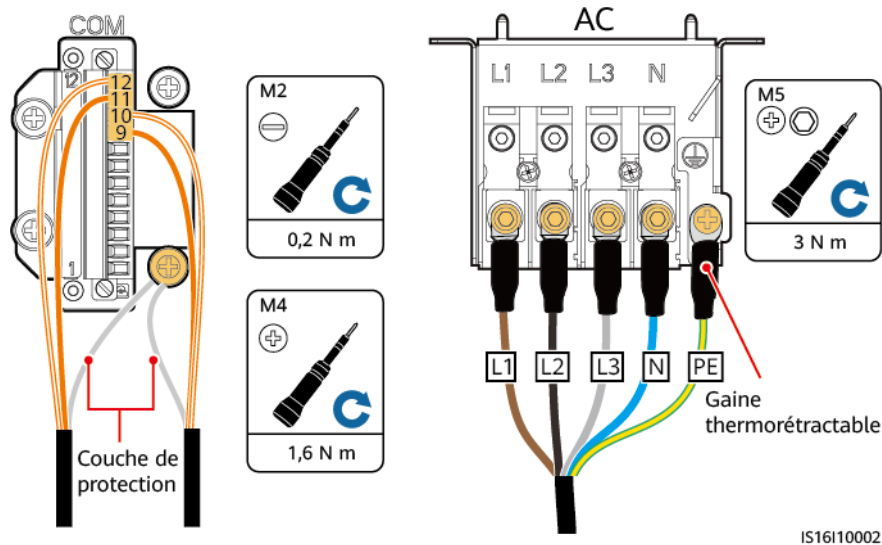
Figure 5-9 Installation des câbles d'alimentation de sortie CA et des câbles de signal
