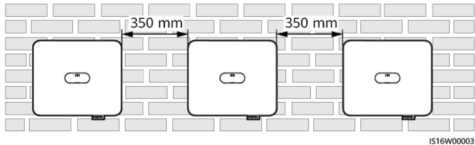
Figure 4-3 Installation horizontale (recommandée)
