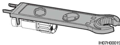
Figure 5-6 Retrait d'un connecteur CC
