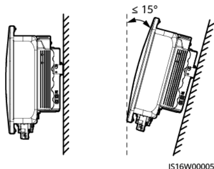
Figure 4-1 Angle d'installation
