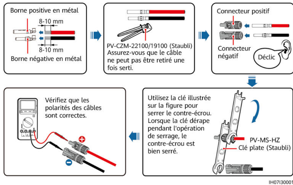
Figure 5-5 Assemblage des connecteurs CC
